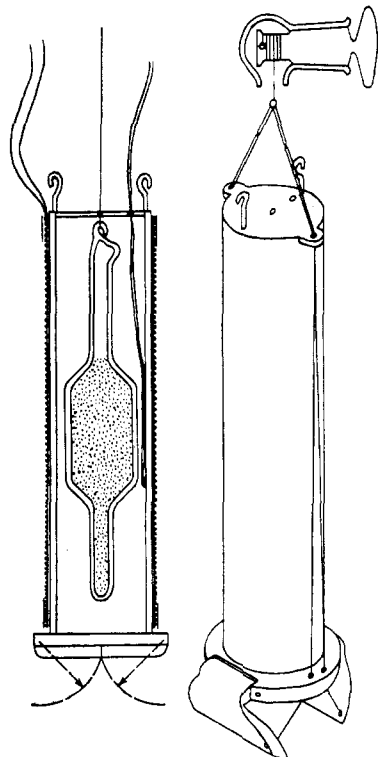
Fig. 2.—Heating unit.
